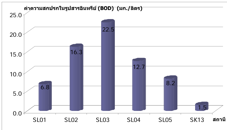
รูปที่ 3 ปริมาณความสกปรกในรูปสารอินทรีย์ (BOD) คลองสำโรง ครั้งที่ 2 ปีงบประมาณ พ.ศ. 2554
