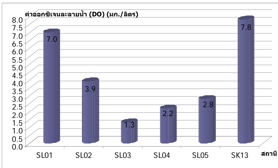
รูปที่ 2 ค่าออกซิเจนละลายน้ำ (DO) คลองสำโรง ครั้งที่ 2 ปีงบประมาณ พ.ศ. 2554
