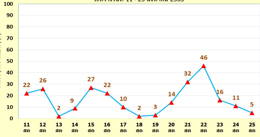
การเปลี่ยนแปลงของจุดความร้อน (Hotspots) บนเกาะสุมาตรา ประเทศอินโดนีเซีย ระหว่างวันที่ 11 - 25 สิงหาคม 2563
