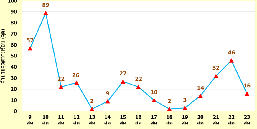
การเปลี่ยนแปลงของจุดความร้อน (Hotspots) บนเกาะสุมาตรา ประเทศอินโดนีเซีย ระหว่างวันที่ 9 - 23 สิงหาคม 2563
