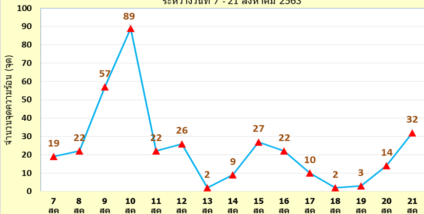
การเปลี่ยนแปลงของจุดความร้อน (Hotspots) บนเกาะสุมาตรา ประเทศอินโดนีเซีย ระหว่างวันที่ 7 - 21 สิงหาคม 2563
