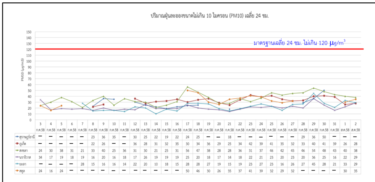
รูปที่ 5 แสดงการเปลี่ยนแปลงของปริมาณฝุ่นละอองขนาดไม่เกิน 10 ไมครอน (PM 10 ) ระหว่างวันที่ 3 ก.ค. – 2 ส.ค. 2558
