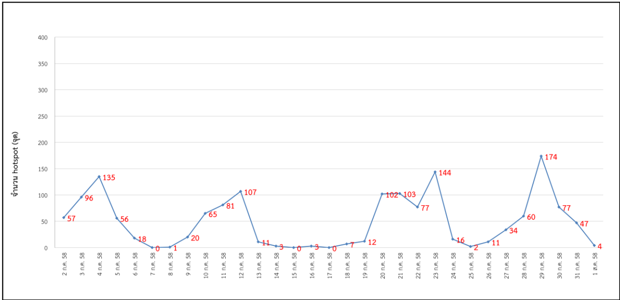
รูปที่ 4 แสดงการเปลี่ยนแปลงของ Hotspot บนเกาะสุมาตรา ระหว่างวันที่ 2 ก.ค. – 1 ส.ค. 2558
