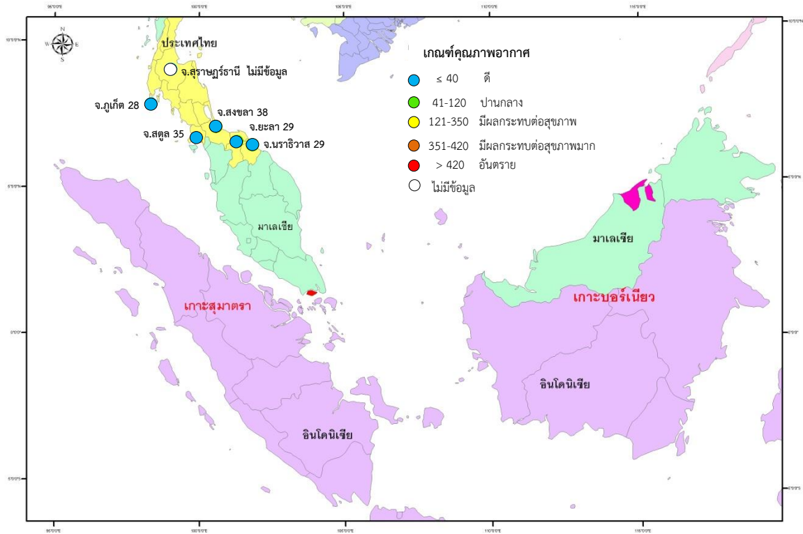
รูปที่ 3 คุณภาพอากาศ วันที่ 2 สิงหาคม 2558
