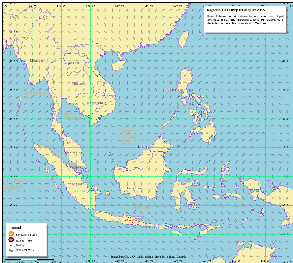
รูปที่ 2 ทิศทางลม เมื่อวันที่ 1 สิงหาคม 2558
