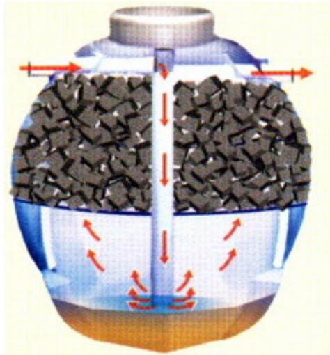
ภาพที่ ๗ ถังกรองไร้อากาศ
