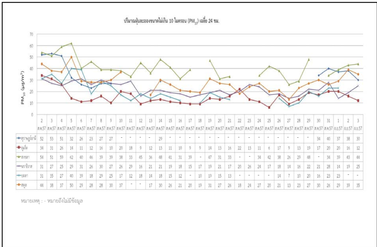
รูปที่ 5 แสดงการเปลี่ยนแปลงของปริมาณฝุ่นละอองขนาดไม่เกิน 10 ไมครอน (PM 10 ) ระหว่างวันที่ 2 ส.ค. - 3 ก.ย. 2557
