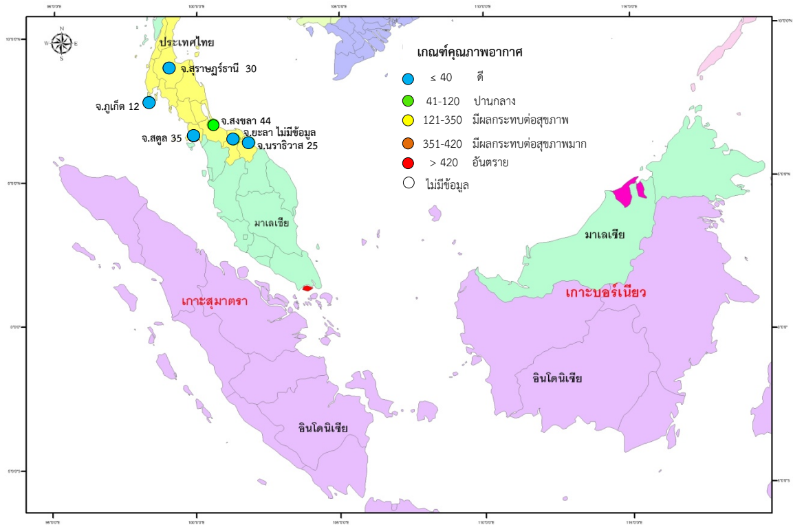
รูปที่ 3 คุณภาพอากาศ วันที่ 3 กันยายน 2557
