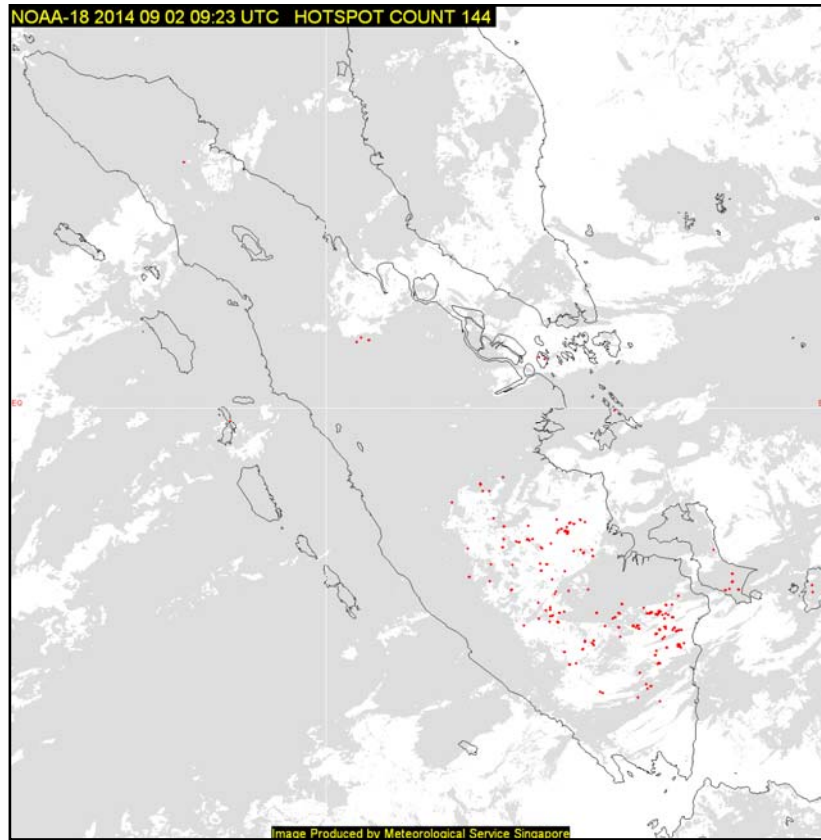
รูปที่ 1 จำนวนจุดที่เกิดไฟไหม้บนเกาะสุมาตรา เมื่อวันที่ 2 กันยายน 2557
