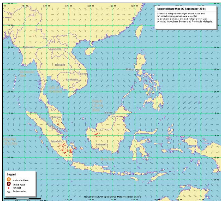
รูปที่ 2 ทิศทางลม เมื่อวันที่ 2 กันยายน 2557
