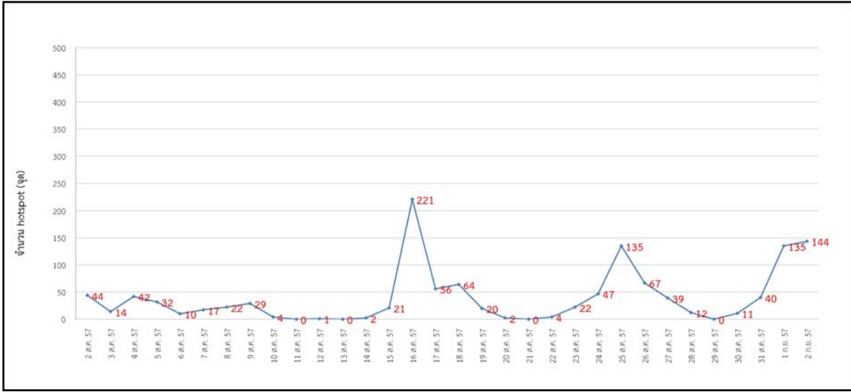
รูปที่ 4 แสดงการเปลี่ยนแปลงของ Hotspot บนเกาะสุมาตรา ระหว่างวันที่ 2 ส.ค. - 2 ก.ย. 2557
