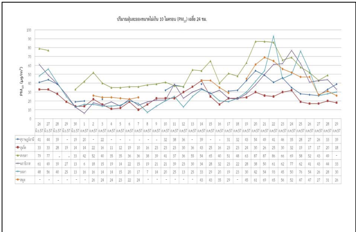
รูปที่ 5 แสดงการเปลี่ยนแปลงของปริมาณฝุ่นละอองขนาดไม่เกิน 10 ไมครอน (PM 10 ) ระหว่างวันที่ 26 มิ.ย. – 29 ก.ค. 2557
