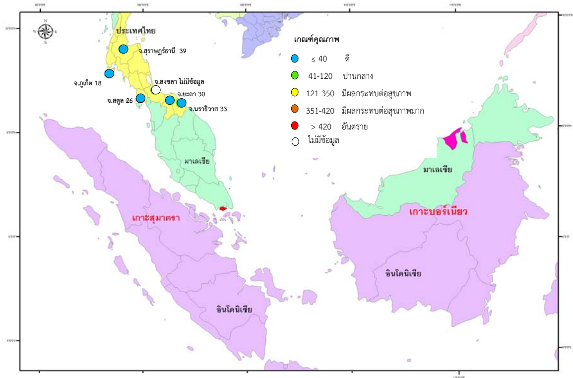
รูปที่ 3 คุณภาพอากาศ วันที่ 29 กรกฎาคม 2557
