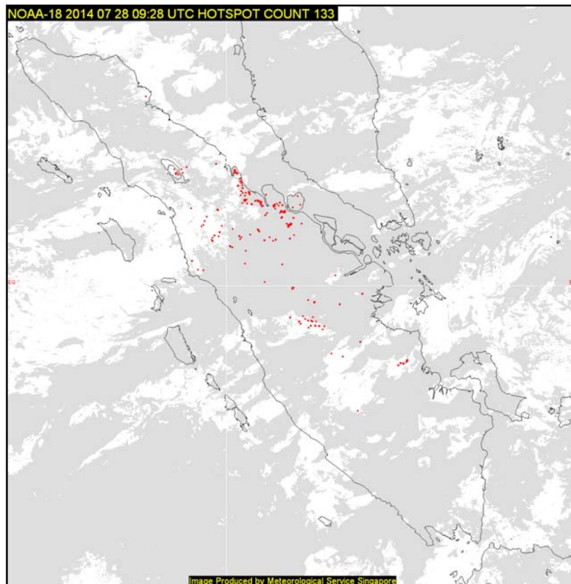
รูปที่ 1 จำนวนจุดที่เกิดไฟไหม้บนเกาะสุมาตรา เมื่อวันที่ 28 กรกฎาคม 2557
