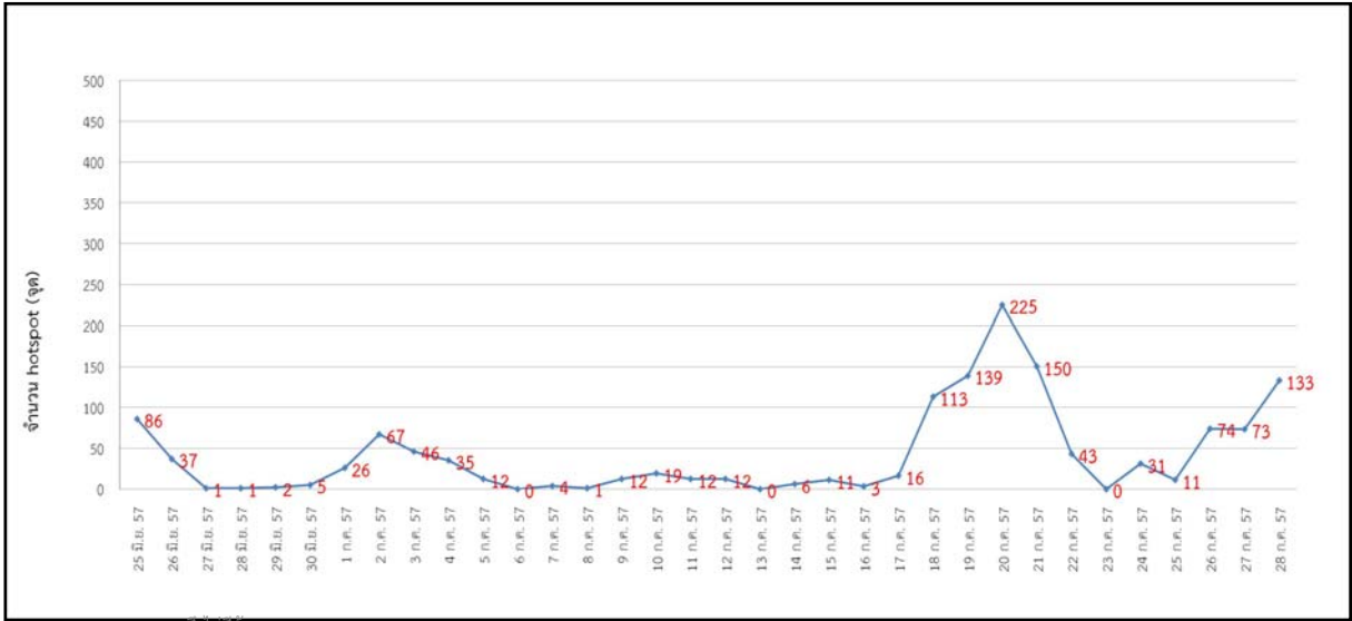
รูปที่ 4 แสดงการเปลี่ยนแปลงของ Hotspot บนเกาะสุมาตรา ระหว่างวันที่ 26 มิ.ย. – 28 ก.ค. 2557
