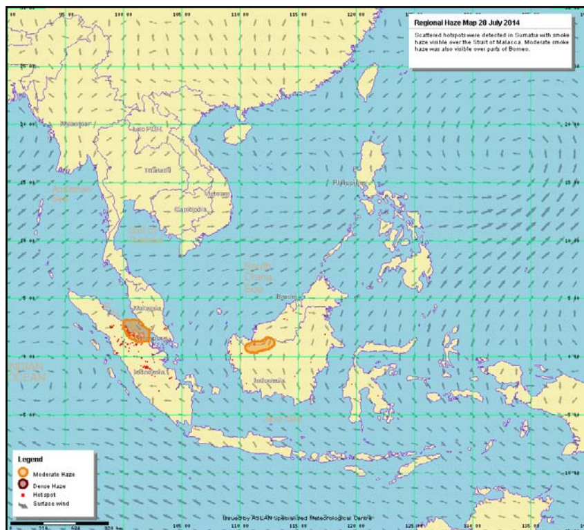
รูปที่ 2 ทิศทางลม เมื่อวันที่ 28 กรกฎาคม 2557
