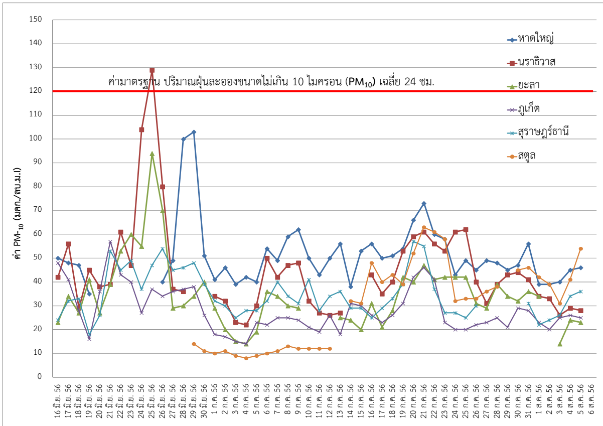
รูปที่ 5 แสดงการเปลี่ยนแปลงของปริมาณฝุ่นละอองขนาดไม่เกิน 10 ไมครอน (PM10) ระหว่างวันที่ 16 มิถุนายน - 5 สิงหาคม 2556
