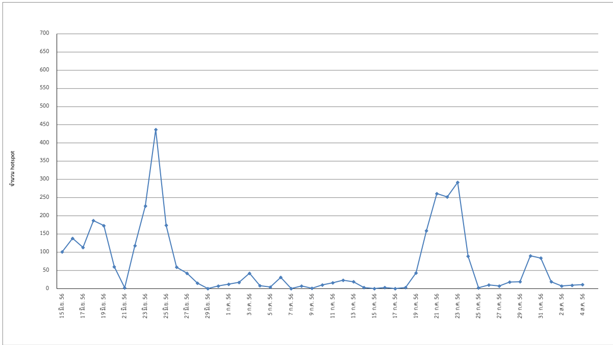
รูปที่ 4 แสดงการเปลี่ยนแปลงของ Hotspot บนเกาะสุมาตรา ระหว่างวันที่ 15 มิถุนายน - 4 สิงหาคม 2556
