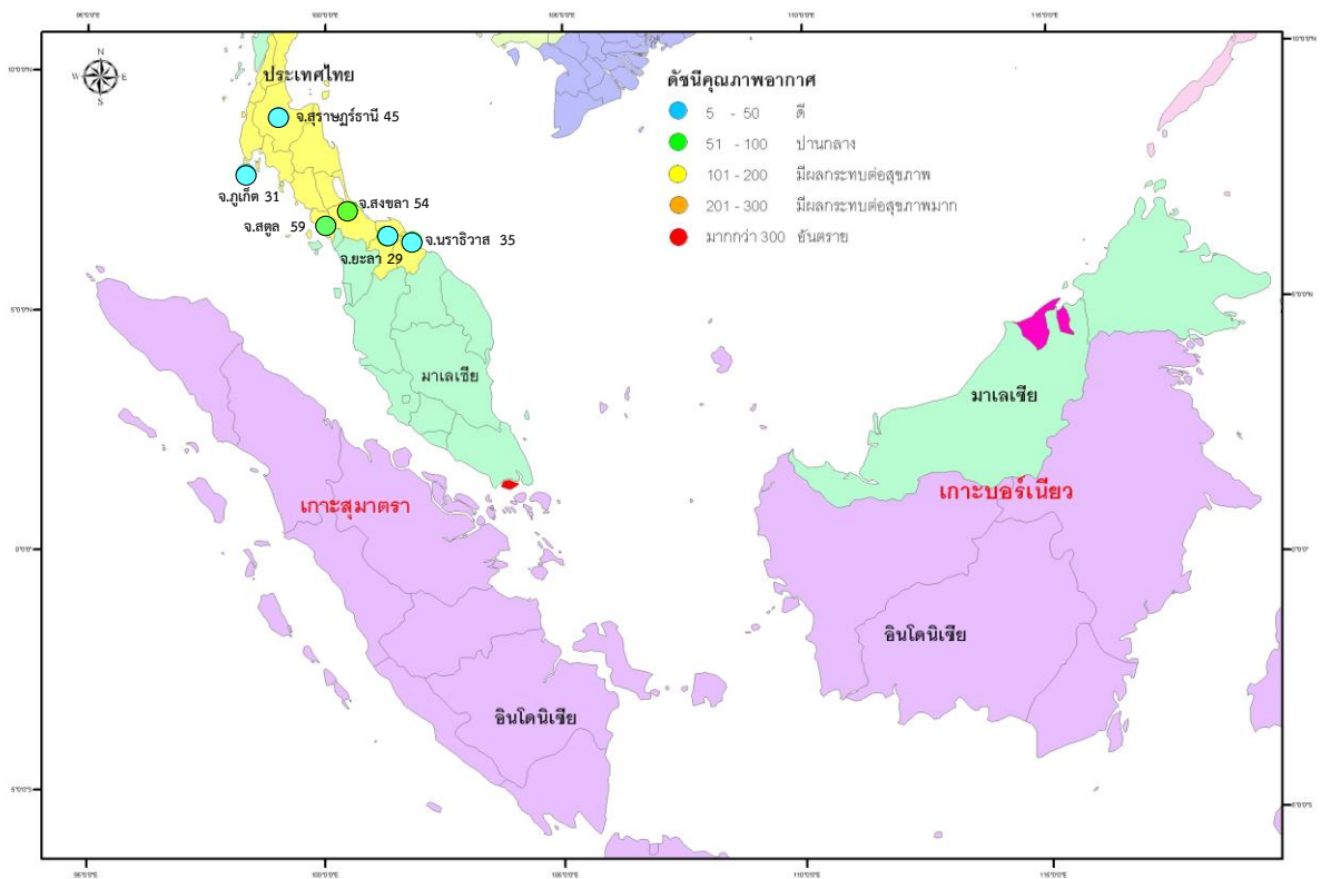
รูปที่ 3 ดัชนีคุณภาพอากาศ วันที่ 5 สิงหาคม 2556
