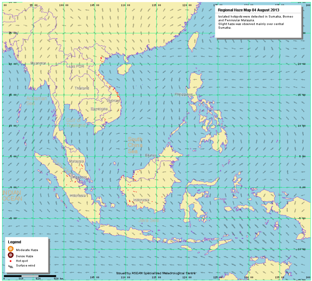
รูปที่ 2 ทิศทางลม เมื่อวันที่ 4 สิงหาคม 2556
