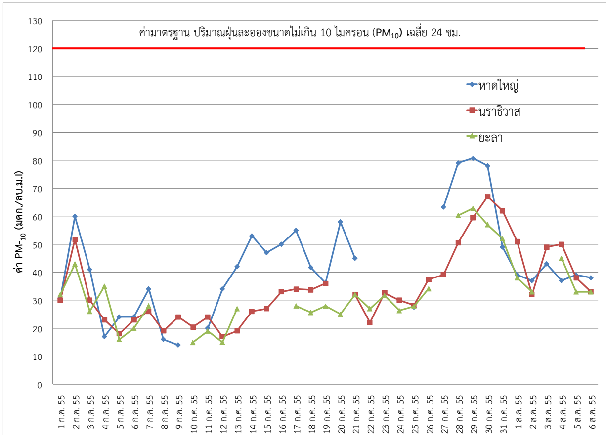
รูปที่ 5 แสดงการเปลี่ยนแปลงของปริมาณฝุ่นละอองขนาดไม่เกิน 10 ไมครอน (PM 10 ) ระหว่างวันที่ 1 กรกฎาคม - 6 สิงหาคม 2555
