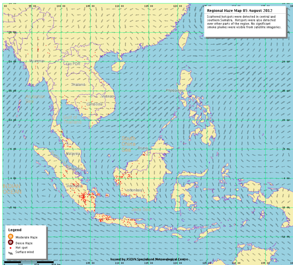
รูปที่ 2 ทิศทางลม เมื่อวันที่ 5 สิงหาคม 2555
