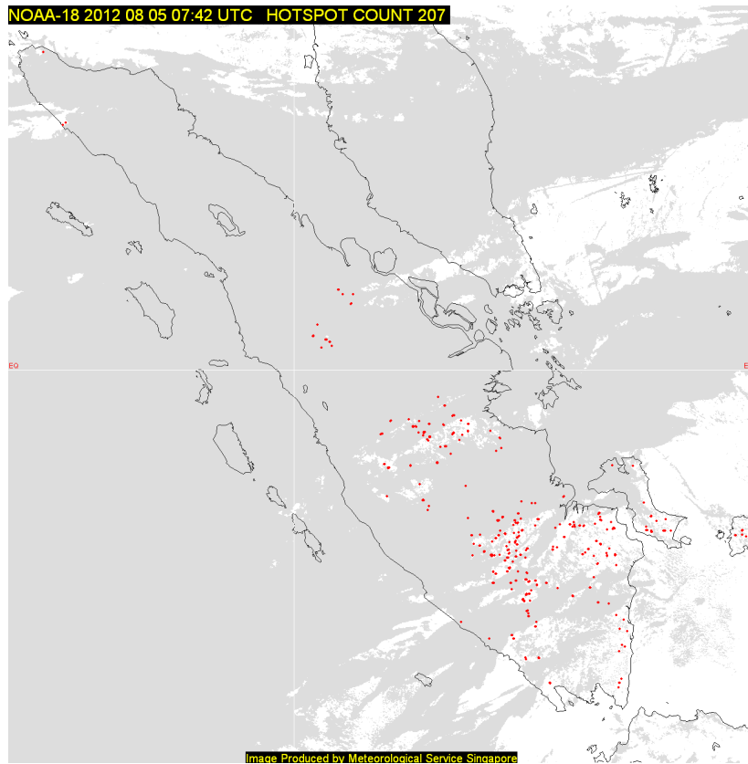
รูปที่ 1 จำนวนจุดที่เกิดไฟไหม้บนเกาะสุมาตรา ประเทศอินโดนีเซีย เมื่อวันที่ วันที่ 5 สิงหาคม 2555
