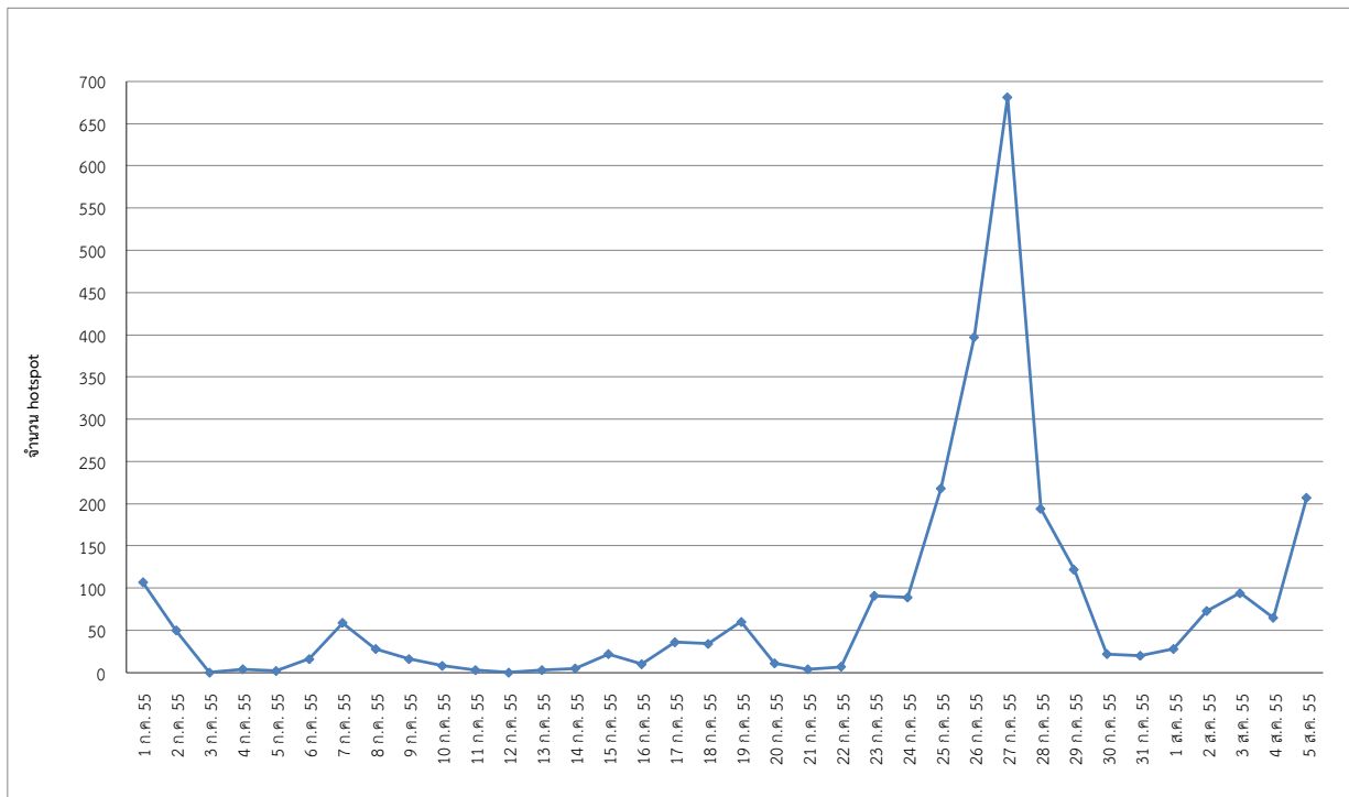
รูปที่ 4 แสดงการเปลี่ยนแปลงของจำนวน Hotspot บนเกาะสุมาตรา ระหว่างวันที่ 1 ก.ค. - 5 ส.ค. 2555
