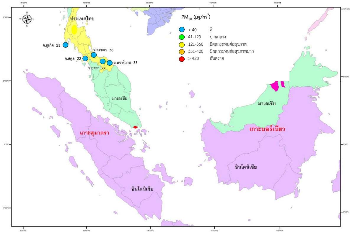
รูปที่ 3 แสดงค่าเฉลี่ยฝุ่นละอองขนาดไม่เกิน 10 ไมครอน ในเวลา 24 ชั่วโมง วันที่ 6 สิงหาคม 2555
