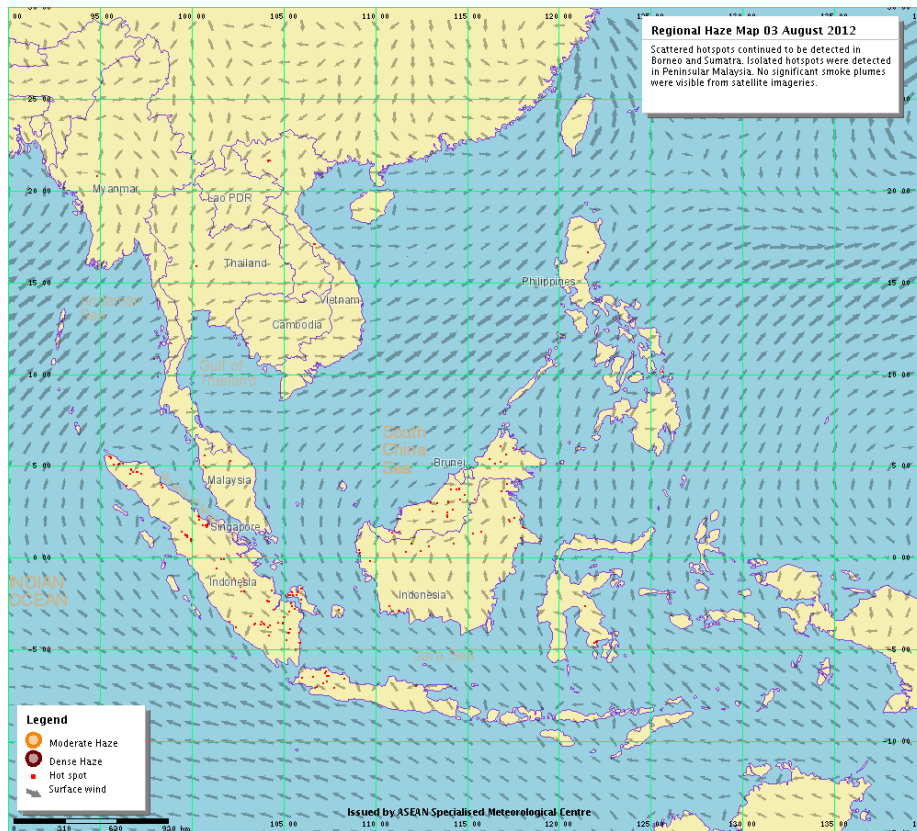
รูปที่ 2 ทิศทางลม เมื่อวันที่ 3 สิงหาคม 2555
