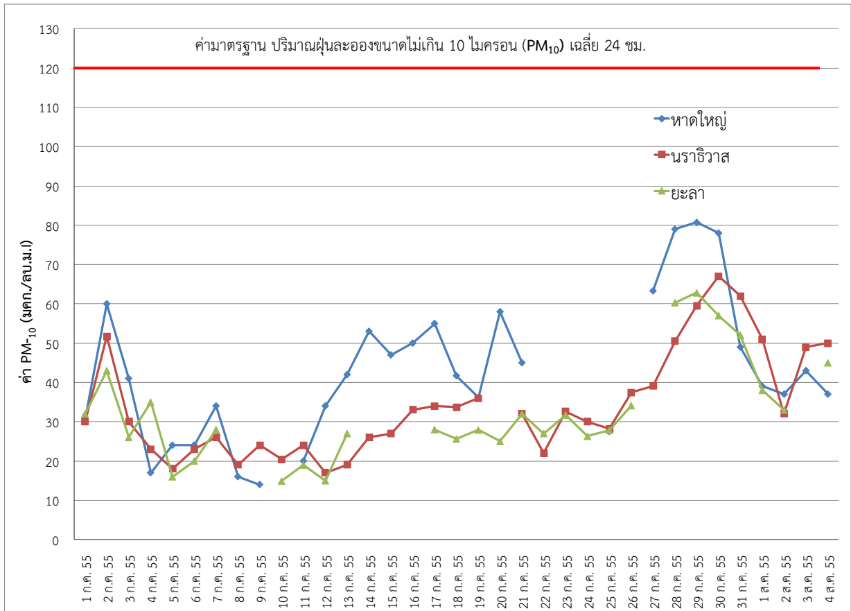
รูปที่ 5 แสดงการเปลี่ยนแปลงของปริมาณฝุ่นละอองขนาดไม่เกิน 10 ไมครอน (PM 10 ) ระหว่างวันที่ 1 กรกฎาคม - 4 สิงหาคม 2555
