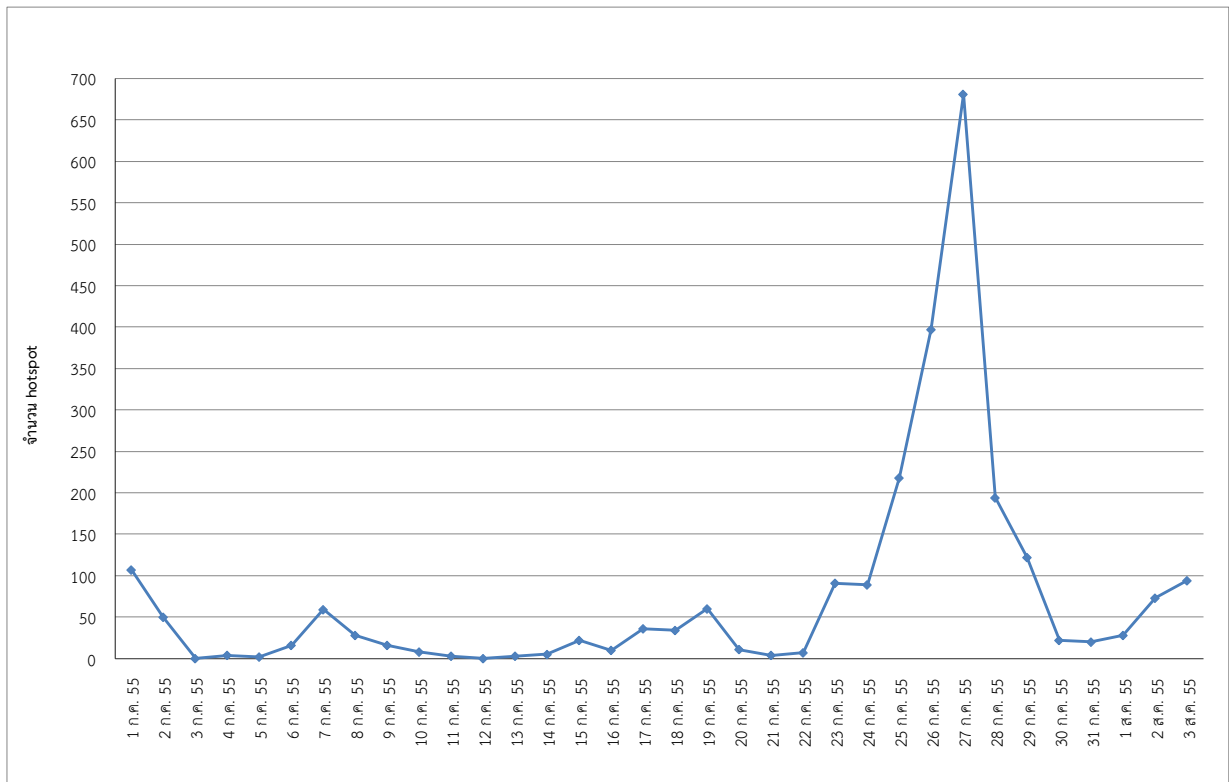
รูปที่ 4 แสดงการเปลี่ยนแปลงของจำนวน Hotspot บนเกาะสุมาตรา ระหว่างวันที่ 1 ก.ค. - 3 ส.ค. 2555
