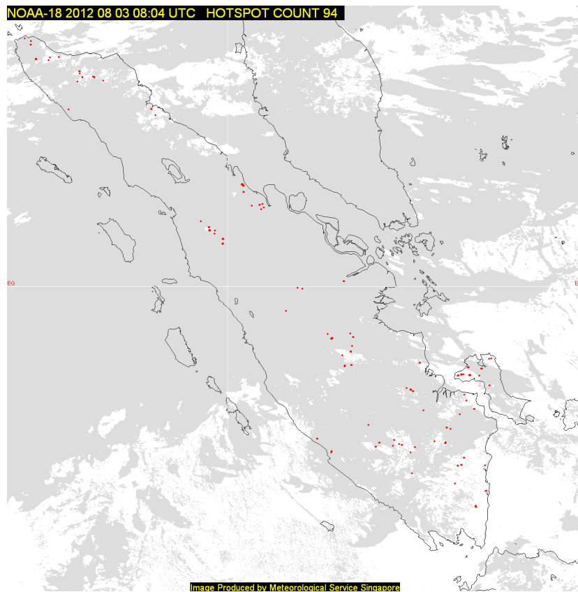
รูปที่ 1 จำนวนจุดที่เกิดไฟไหม้บนเกาะสุมาตรา ประเทศอินโดนีเซีย เมื่อวันที่ วันที่ 3 สิงหาคม 2555
