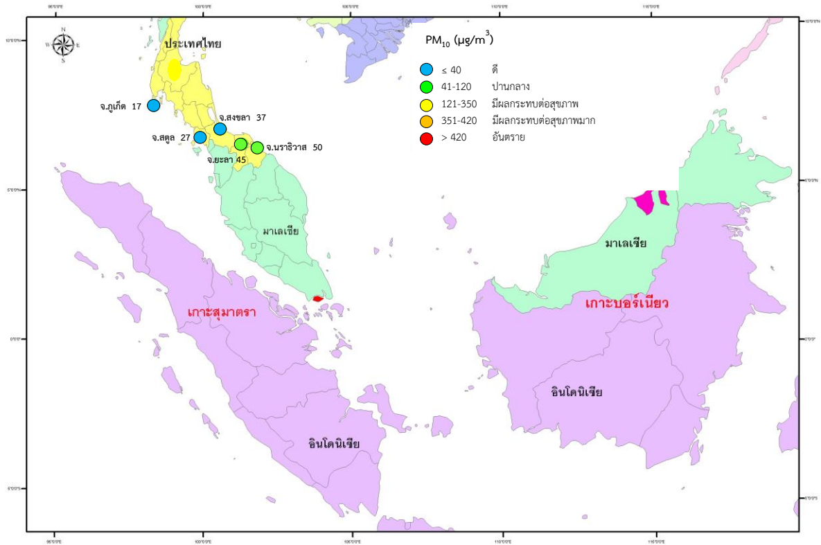
รูปที่ 3 แสดงค่าเฉลี่ยฝุ่นละอองขนาดเล็กไม่เกิน 10 ไมครอน ในเวลา 24 ชั่วโมง วันที่ 4 สิงหาคม 2555 (จังหวัดสตูล เป็นข้อมูลวันที่ 1 สิงหาคม 2555 และจังหวัดภูเก็ต เป็นข้อมูลวันที่ 3 สิงหาคม 2555)
