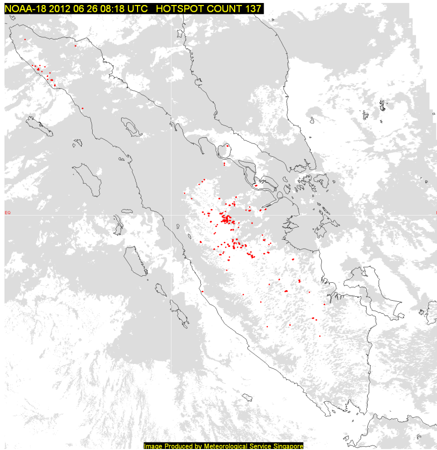
รูปที่ 1 จำนวนจุดที่เกิดไฟไหม้บนเกาะสุมาตรา ประเทศอินโดนีเซีย เมื่อวันที่ 26 มิถุนายน 2555
