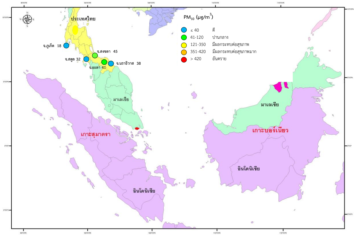
รูปที่ 3 แสดงค่าเฉลี่ยฝุ่นละอองขนาดไม่เกิน 10 ไมครอน ในเวลา 24 ชั่วโมง วันที่ 27 มิถุนายน 2555
