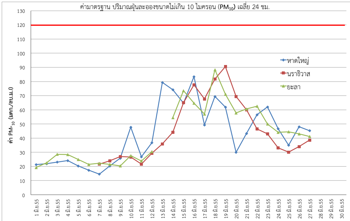
รูปที่ 5 แสดงการเปลี่ยนแปลงของปริมาณฝุ่นละอองขนาดไม่เกิน 10 ไมครอน (PM 10 ) ระหว่างวันที่ 1 - 27 มิถุนายน 2555
