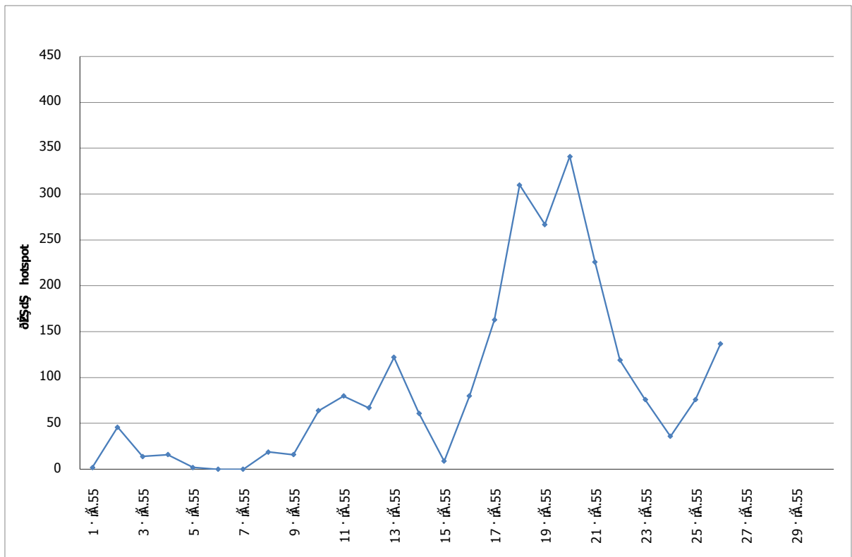
รูปที่ 4 แสดงการเปลี่ยนแปลงของจำนวน Hotspot บนเกาะสุมาตรา ระหว่างวันที่ 1-26 มิถุนายน 2555
